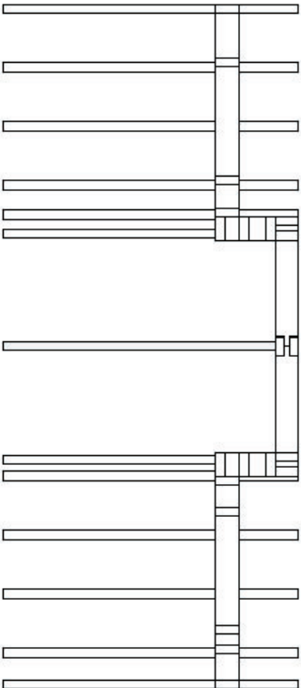
Planbillede af bjælkelag og stolpekonstruktion 1:20
