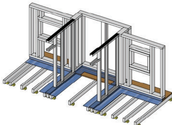
Vægkonstruktionen samles og rejses
